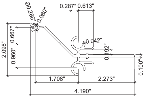
26 // 6063-T6 UNIMATE CENTER MATE OPTION 3
