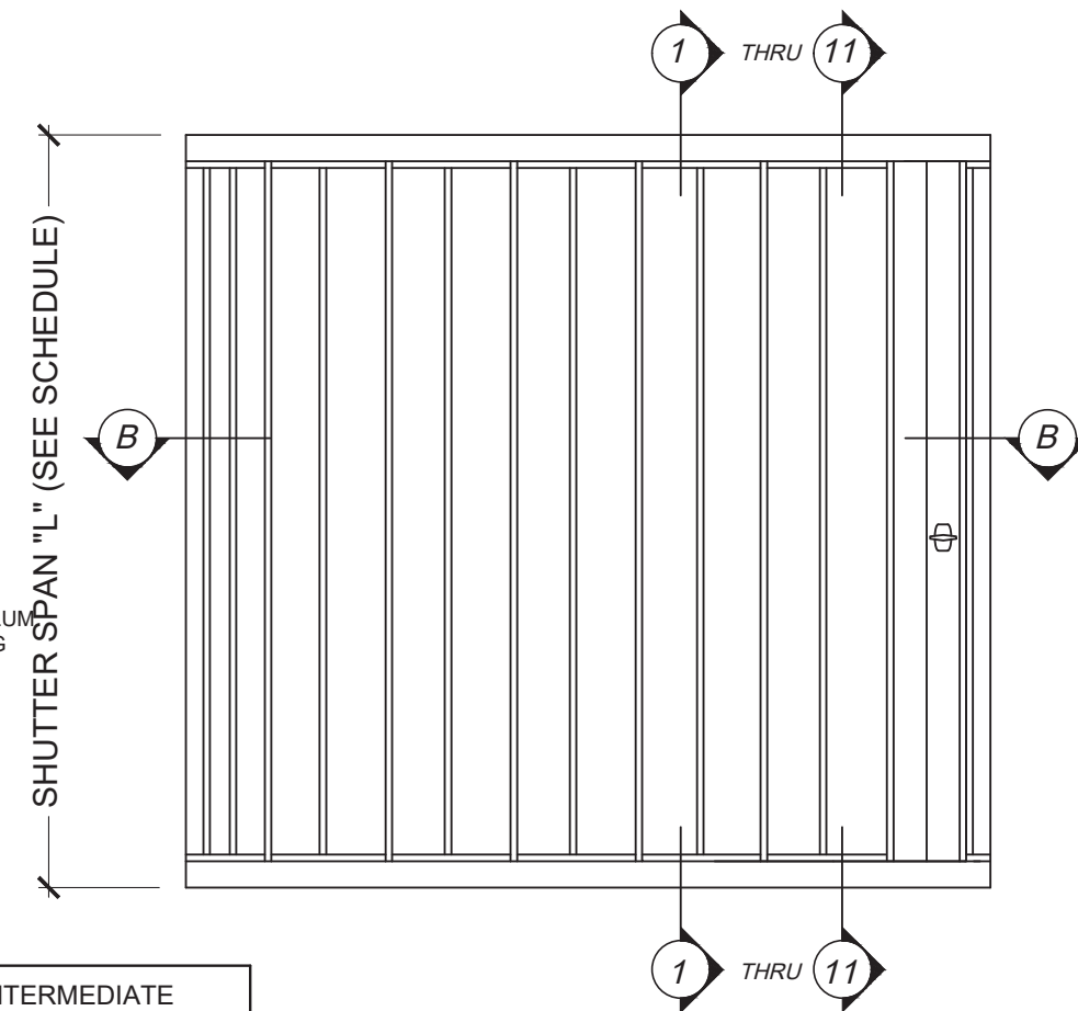
ELEVATION OPTION 2
